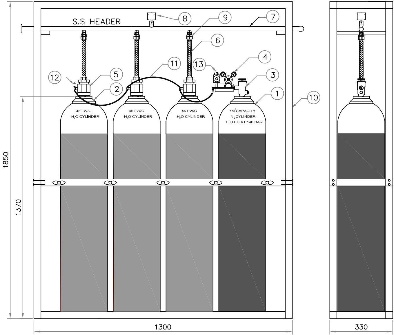
ELEVATION
